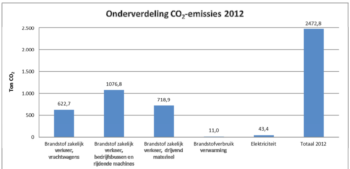
Figuur 5 en 6: onderverdeling CO 2 -emissies, 2012
